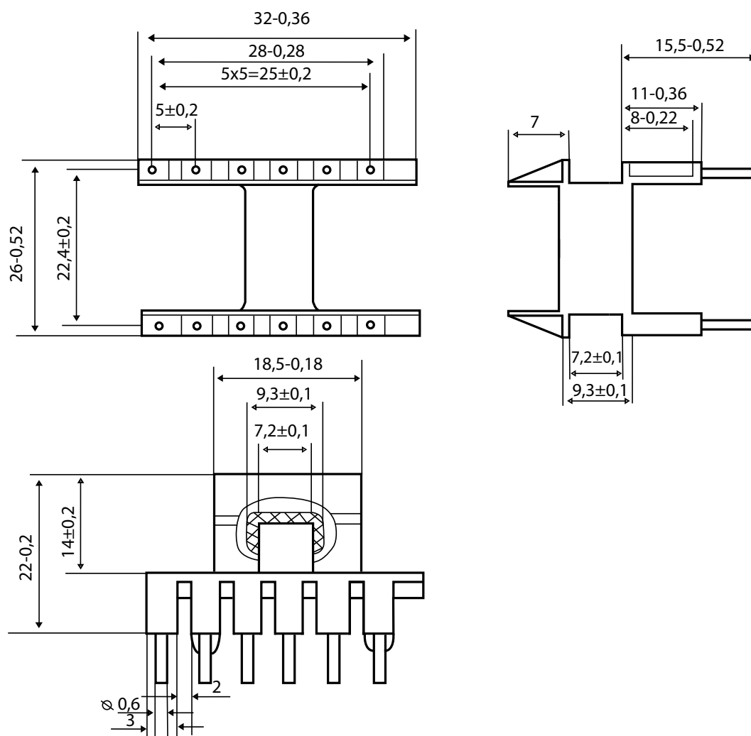
Габаритный чертеж
